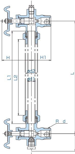
■GVS-BP-R-14 ボールチャッキ付 プラグ弁付
