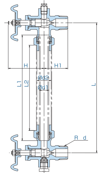
■GVS-P-R-14 プラグ弁付
